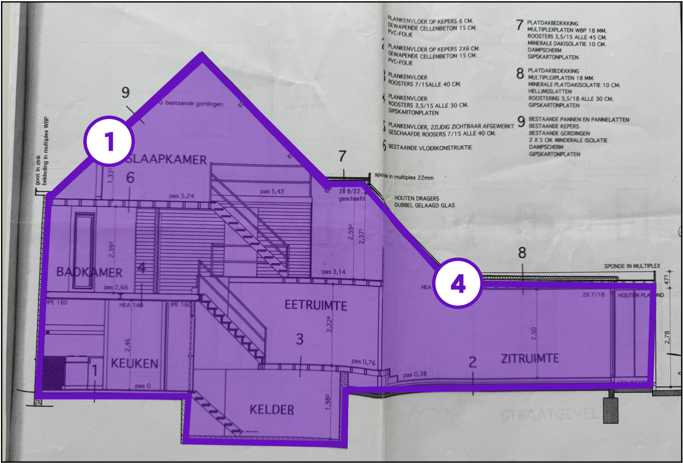
Legende van plan 1.12: Doorsnede kopie
