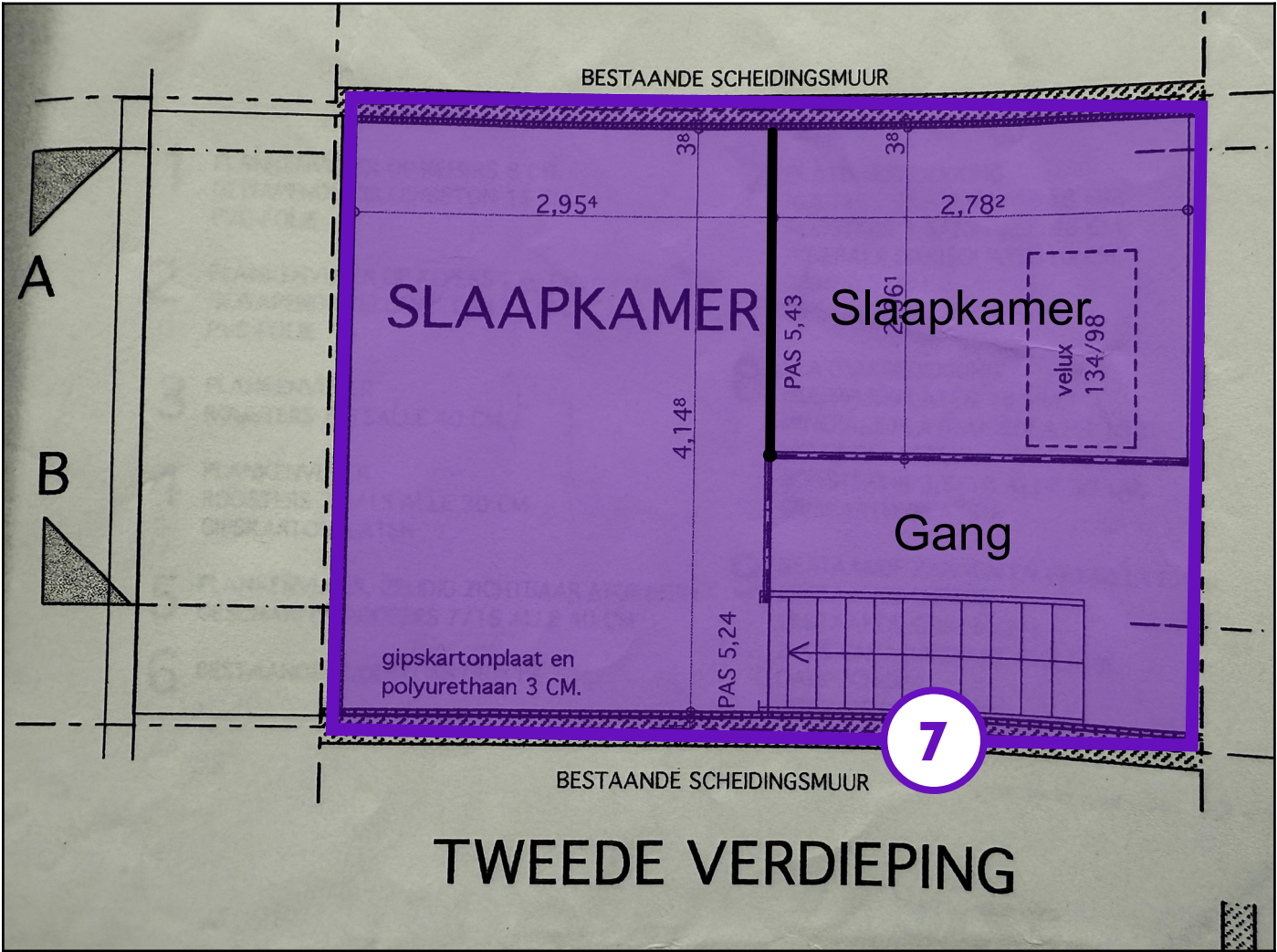
Legende van plan 1.9: 2de verdieping muren
