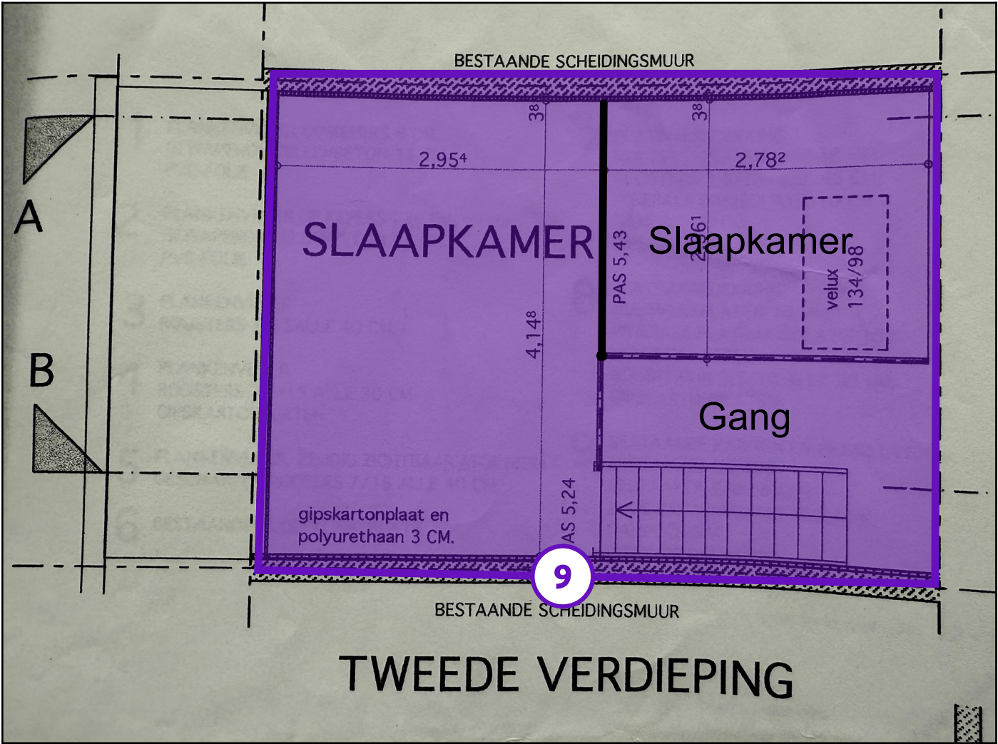
Legende van plan 1.10: 2de verdieping plafonds
